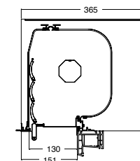
PUKA Plus RA 300 mit 130er Öffnung (Rolladen im Raffstore-System)
